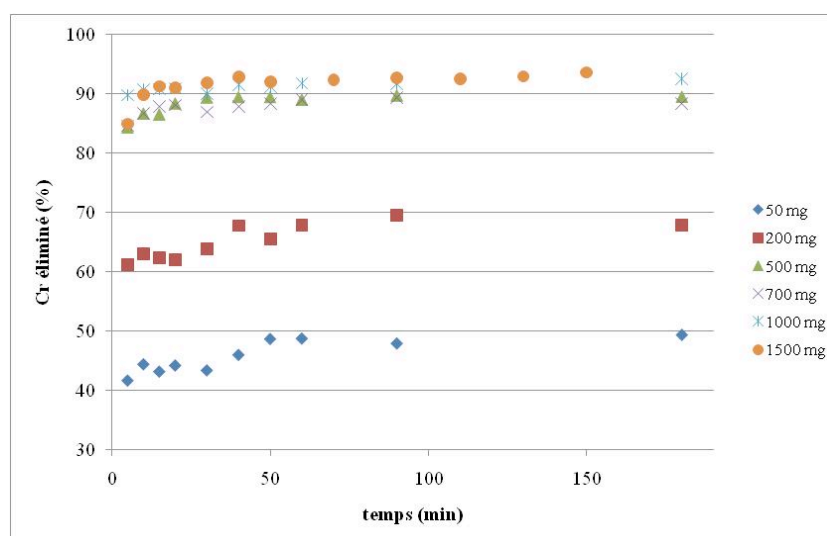
Figure 4 : Cinétiques de la boue V1 pour différentes masses pour [\text{Cr}_2\text{O}_7^{2-}] = 30 \text{ mg.L}^{-1}
