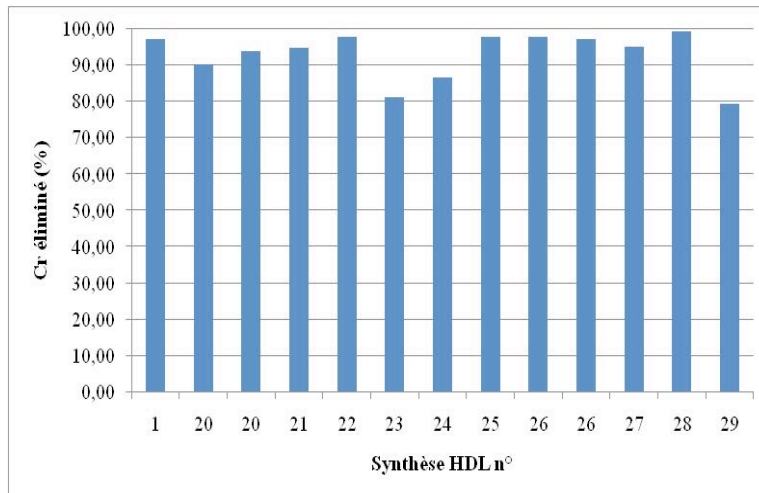
Figure 8 : Taux d'adsorption
