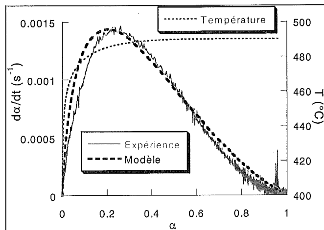
Figure 6. Vitesse expérimentale à 490°C et pour P_{H_2O}=2,5 \text{ hPa} et vitesse calculée à l'aide du modèle non isotherme
