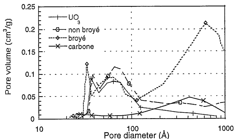
Figure 2 : Courbes de répartition du volume poreux en fonction du diamètre des pores du carbone, trioxyde d'uranium, ( \text{UO}_3+3\text{C} ) et ( \text{UO}_3+3\text{C} ) broyé
