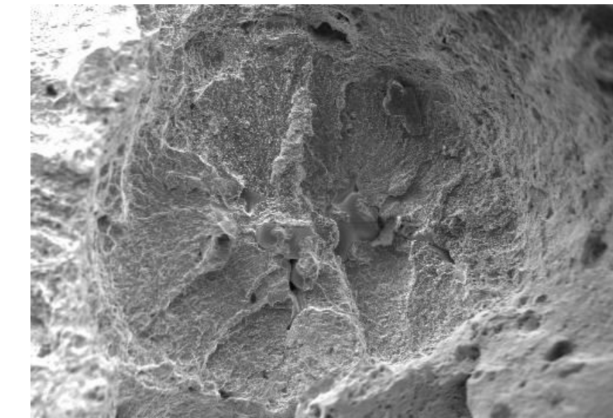
Oeil de poisson sur une surface de rupture d'un acier moulé
