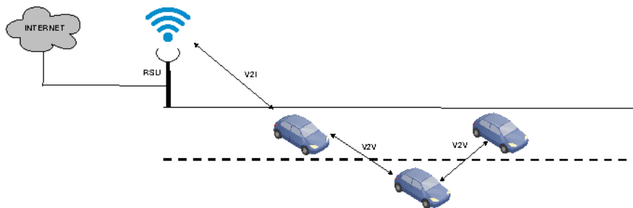
Fig. 1: DSRC Example
