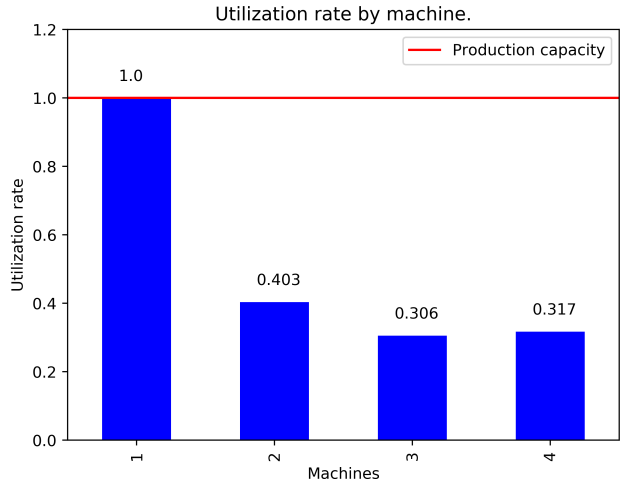
(d) Machine utilization rates for \gamma = 6 .
