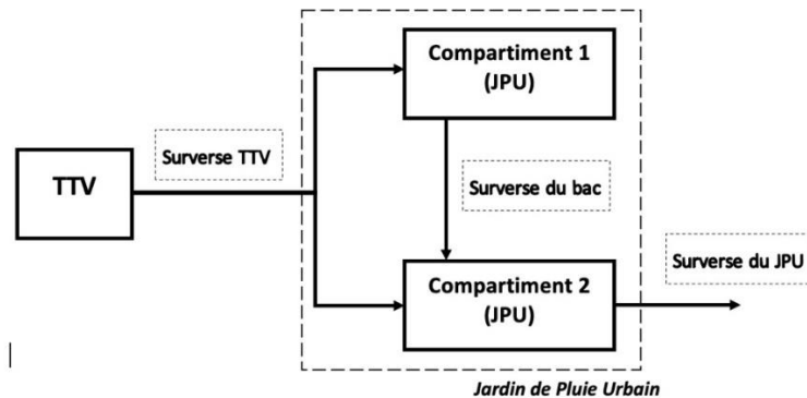
Figure 15 : Proposition de modélisation du dispositif TTV+JPU
