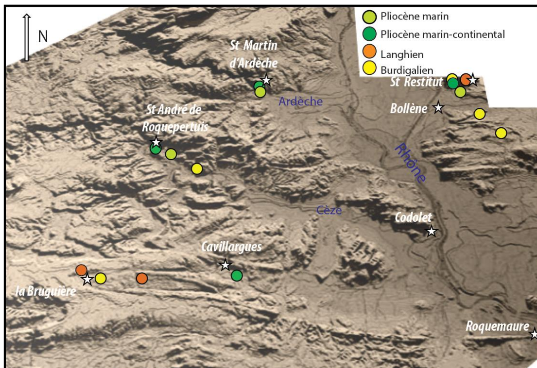
fig. 5 - Dépôts extérieurs régionaux du Néogène encadrant le site des gorges de l'Ardèche
