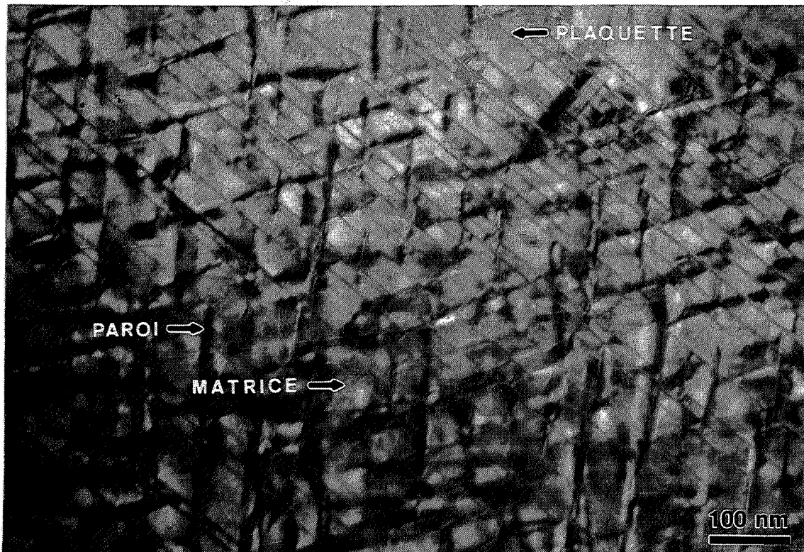
figure IV.1: Microstructure cellulaire de l'échantillon trempé à partir de 910°C. Image en champ clair; axe de zone [11\bar{2}0] .
