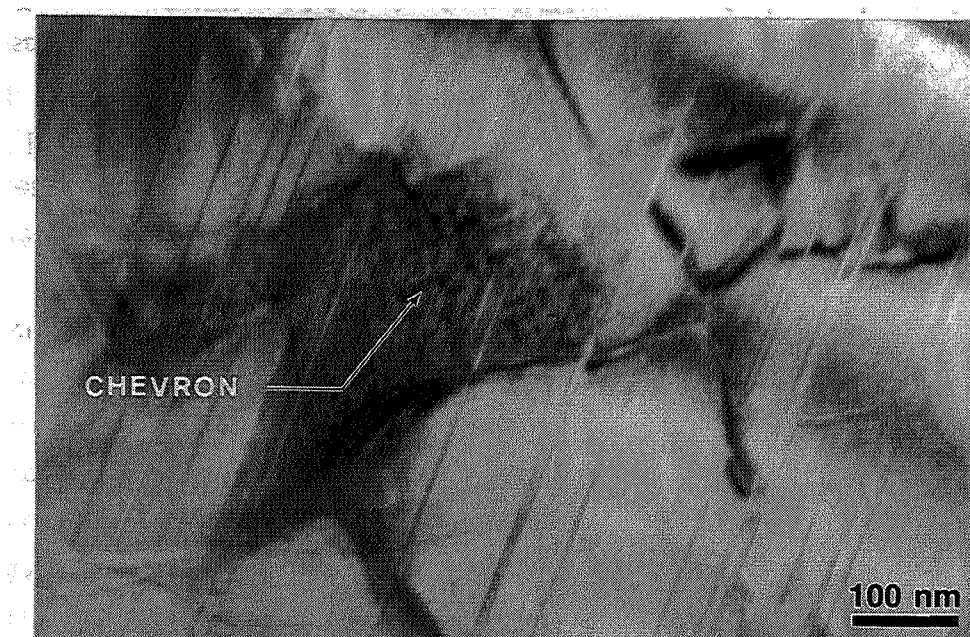
figure V.4: Contraste des chevrons en axe de zone [11\bar{2}0]
