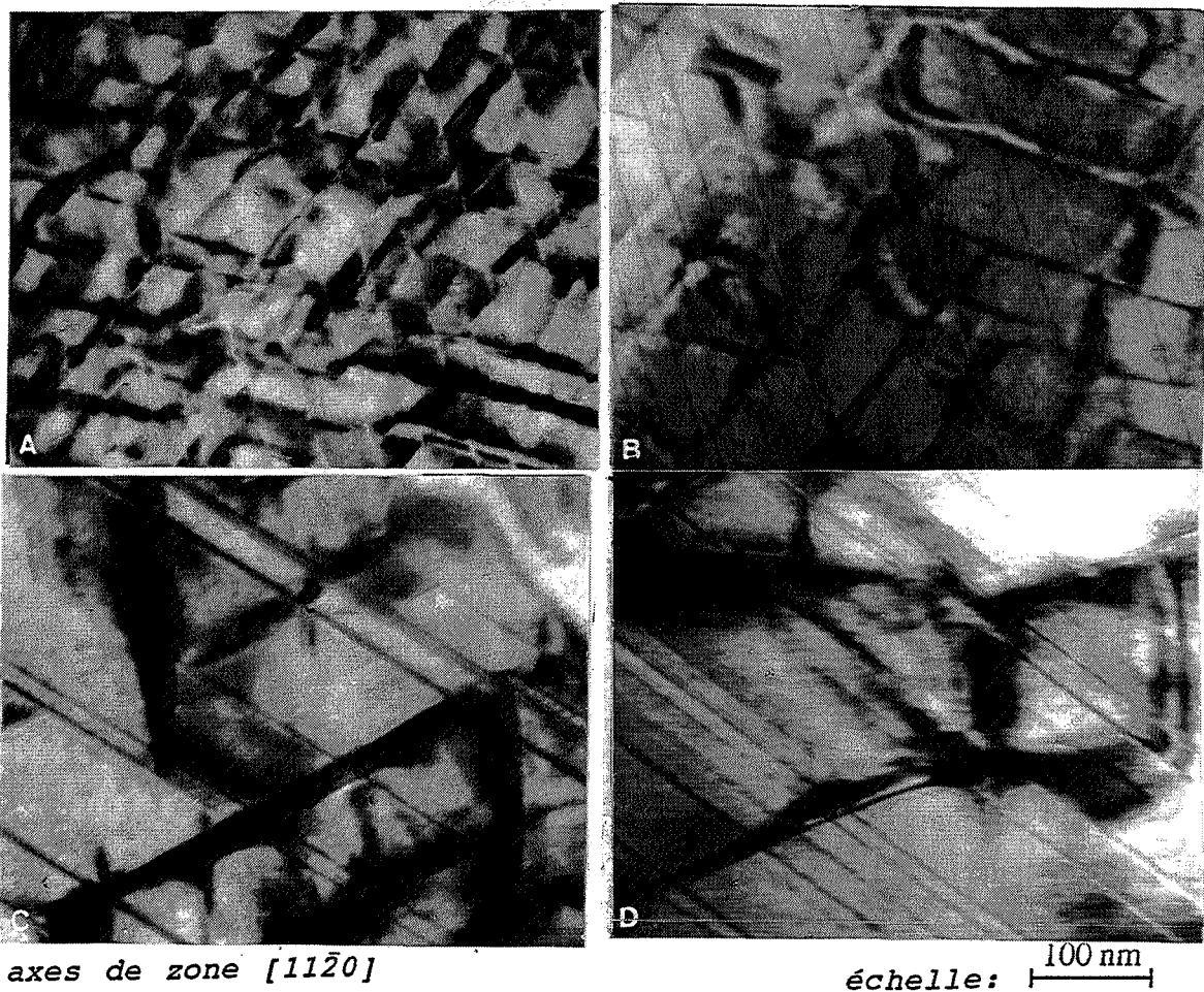
figure IV.15: Evolution de la microstructure cellulaire en fonction de la température. Echantillons trempés à partir de:
