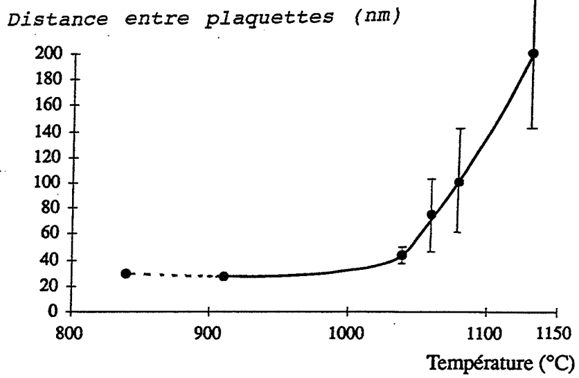
figure IV.17: Distance entre plaquettes en fonction de la température (nuance Récoma). Temps de maintien de 10 min, sauf pour la température de 1040°C (2 min)
