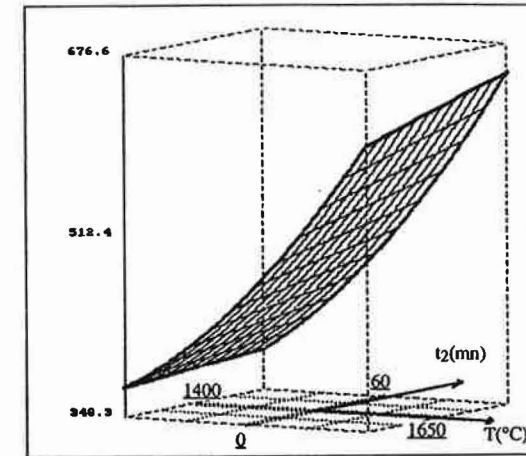
Fig VI-21 : Courbes d'isoréponses précisant l'évolution de la résistance à la flexion (en MPa) entre 1400 ^{\circ}\text{C} et 1650 ^{\circ}\text{C} (les variables fixées sont t_1 = 30 mn et p = 25 MPa). (1) : composition à 0,04 mol% MgO (2) : composition à 3,3 mol% MgO
