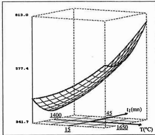
Fig VI-20 : Courbes d'isoréponses précisant l'évolution de la résistance à la flexion (en MPa) entre 1400 ^{\circ}\text{C} et 1650 ^{\circ}\text{C} (les variables fixées sont t_2 = 30 mn et p = 25 MPa). (1) : composition à 0,04 mol% MgO (2) : composition à 3,3 mol% MgO
