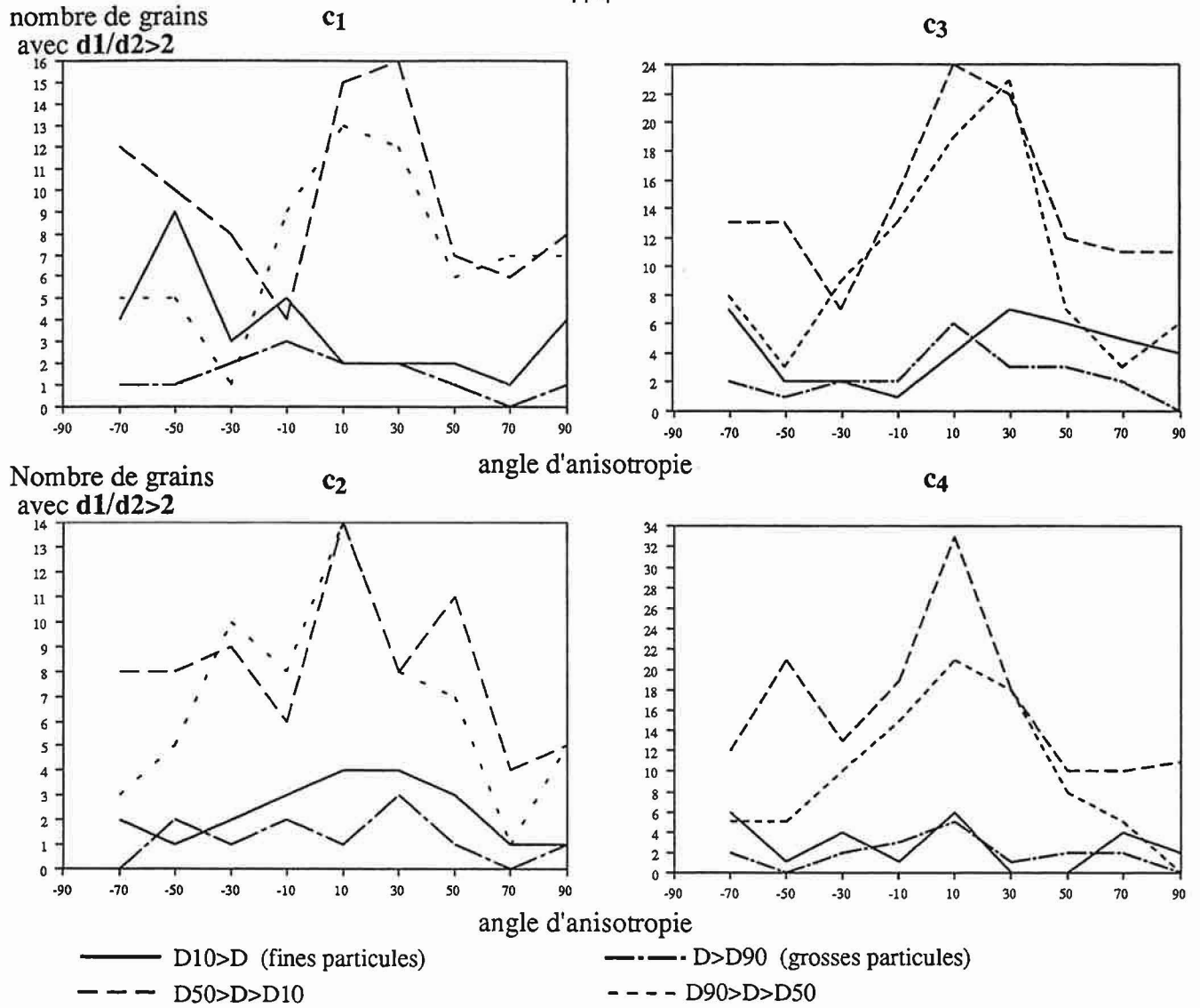
Fig V-13 : Nombre de grains allongés par taille en fonction de l'angle d'anisotropie dans le cas du frittage sous charge.
