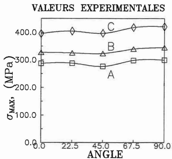
LAMINAGE A FROID ε=2.5
