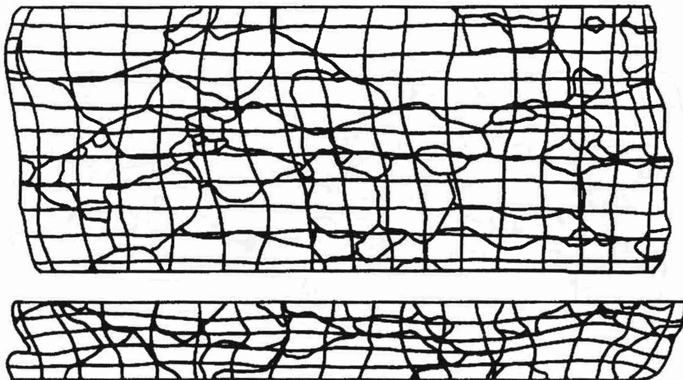
Figure V.3 : Evolution de la forme des grains avant et après déformation, \epsilon = 0,48 .
