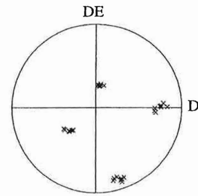
Grains de 11 à 18 ( S^+ )
