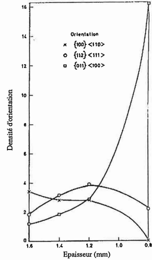
(b) RECRISTALLISE
