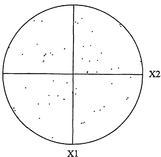
Figure V.11 : Figure des pôles \{111\} obtenue par ECP ; échantillon d'orientation initiale (111)[11\bar{2}] , déformé à \epsilon = 0,25 et recuit 10 heures à 400 °C.
