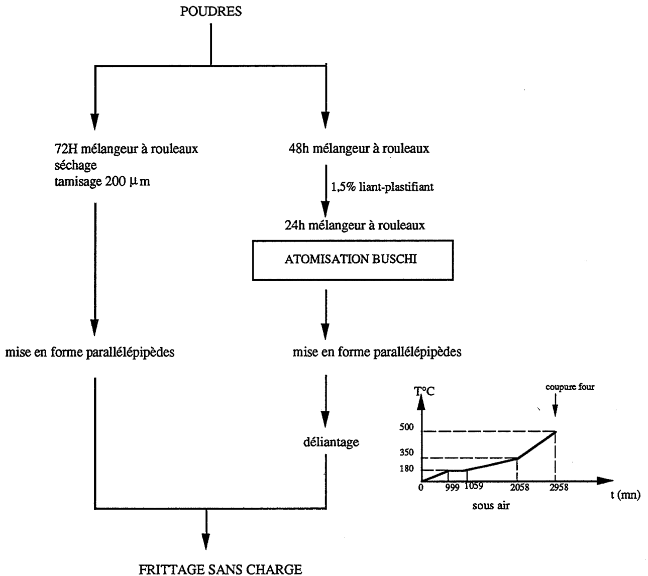
Figure 2-5 : Procédé d'élaboration des échantillons.
