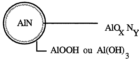
Fig. I.20 Description d'un grain de nitruure d'aluminium
